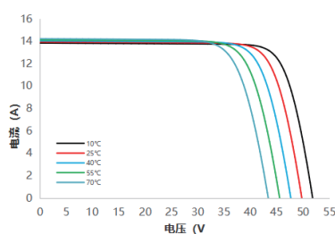
电流-电压曲线 SS8-72HD-545M-T
