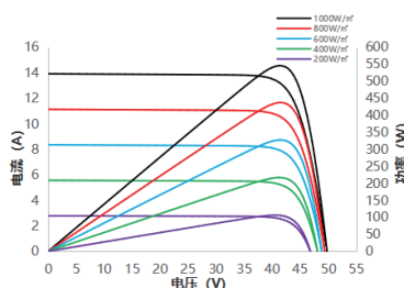
电流/功率-电压曲线 SS8-72HD-545M-T
